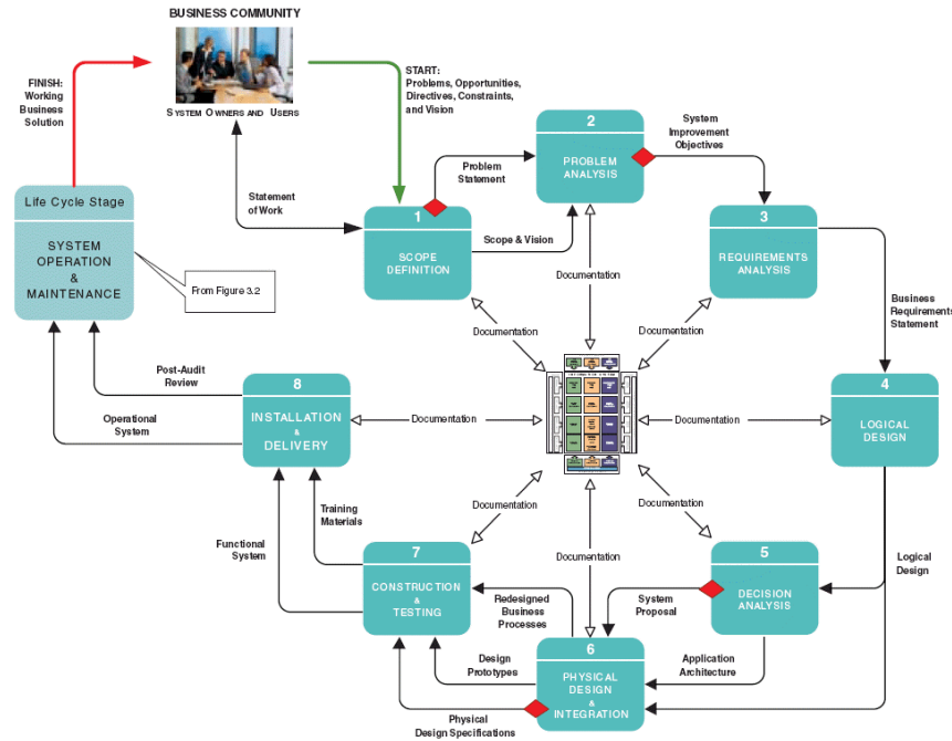
Gambar 3.1. – Metode Pengembangan Sistem FAST
