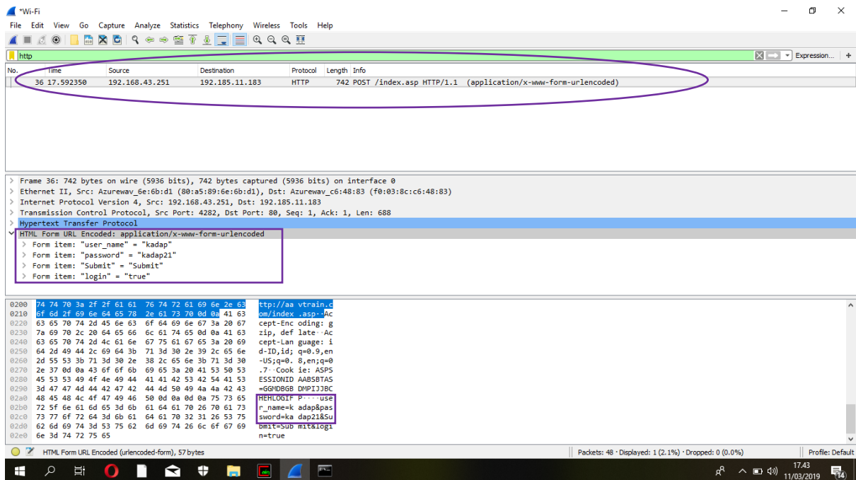
Gambar 1. Hasil trafik menggunakan wireshark
